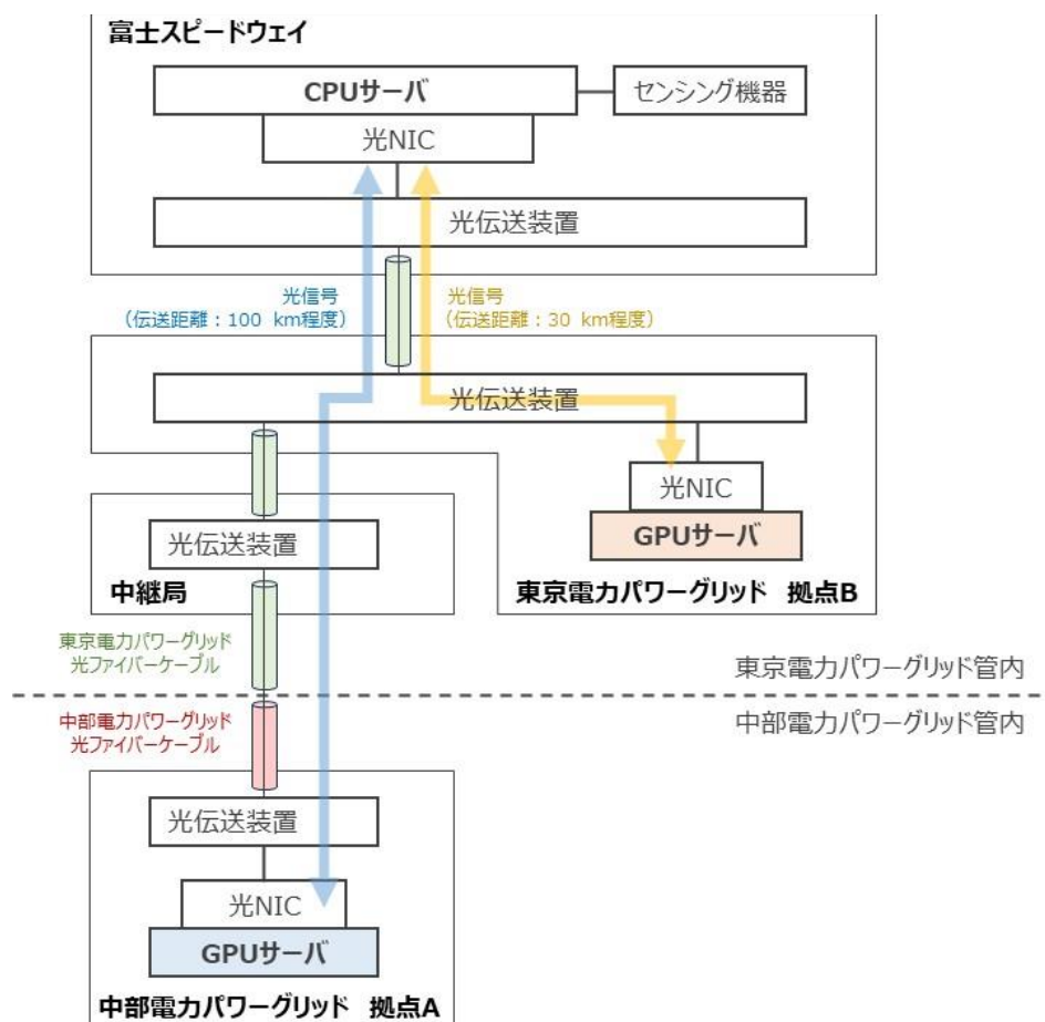
実証実験のインフラ構成図
